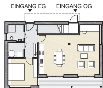
ERDGESCHOSS
